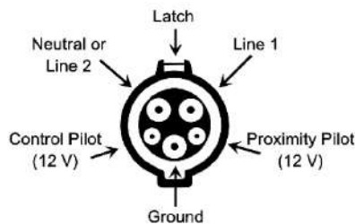
Figura 7 - Connettore J1772
