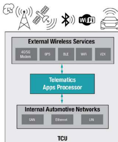
Figura 6 – Il controllo telematico collega il veicolo al mondo esterno.
